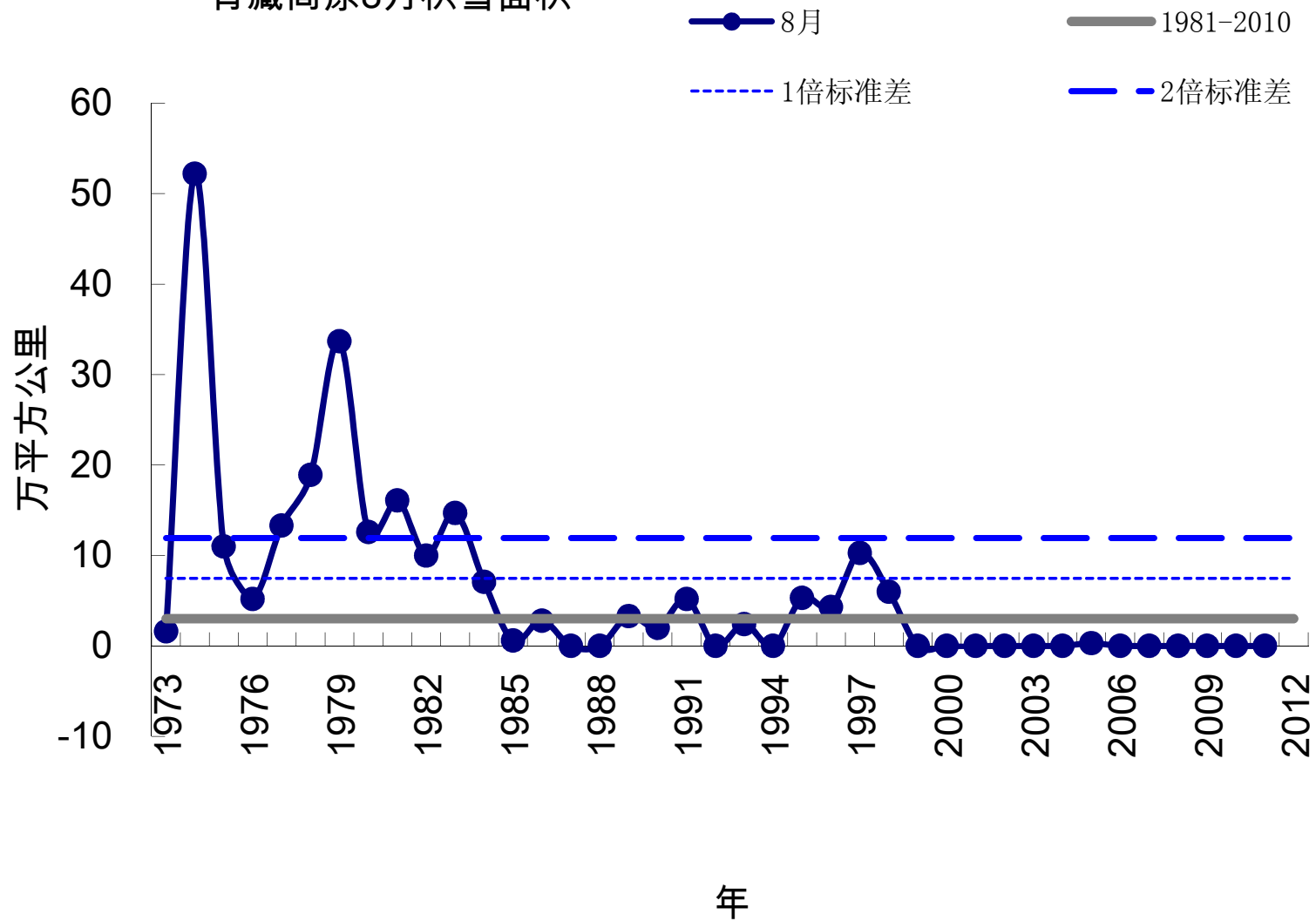
青藏高原8月积雪面积
