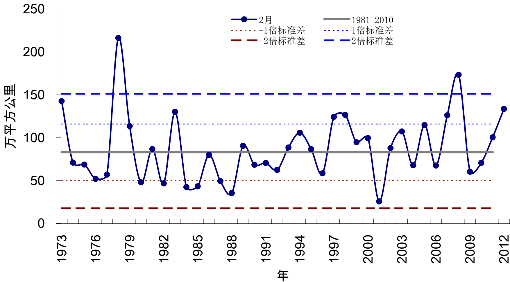
青藏高原2月积雪面积
