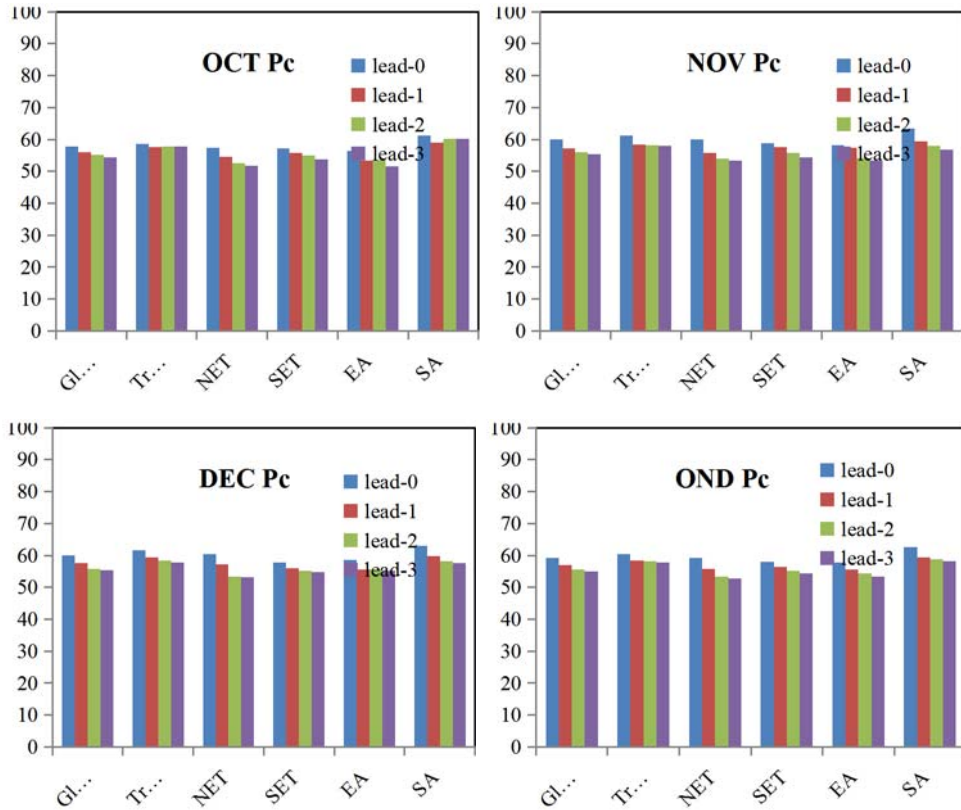
图 16 DERF2.0 在不同 lead time 起报的 10 月、11 月、12 月和第 4 季度的降水 (prec) 的距平符号一致率的不同地区的多年平均
