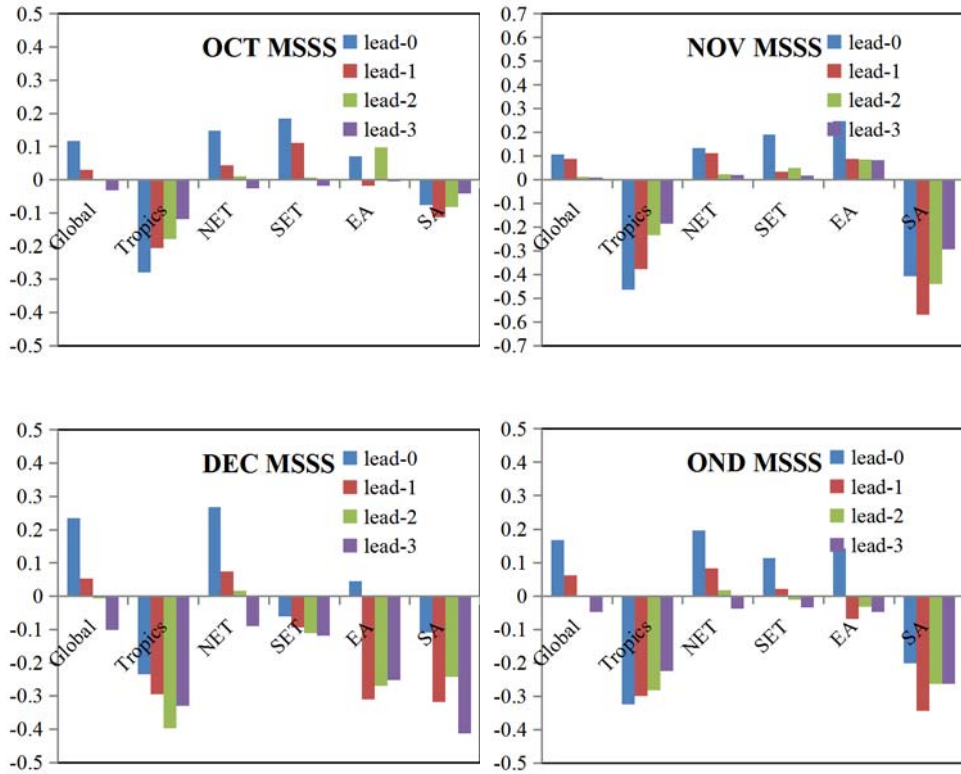
图 12 DERF2.0 在不同 lead time 起报的 10 月、11 月、12 月和第 4 季度的 2m 温度 (t2m) 的平均方差技巧 (MSSS) 在不同地区的平均
