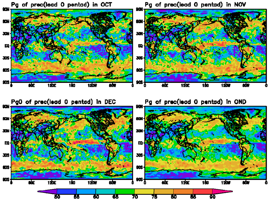
图 19 DERF2.0 超前 0 候起报的的全球 10 月、11 月、12 月和第 4 季度的降水 (prec) 的 Pg 评分多年平均分布
