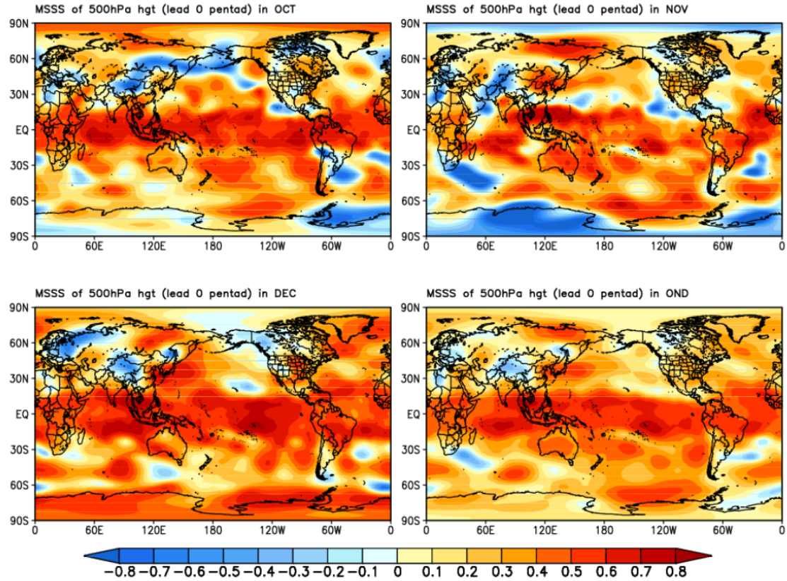
图 28 DERF2.0 超前 0 候起报的全球 10 月、11 月、12 月和第 4 季度的 500hPa 位势高度 (HGT) 的平均方差技巧 (MSSS) 分布
