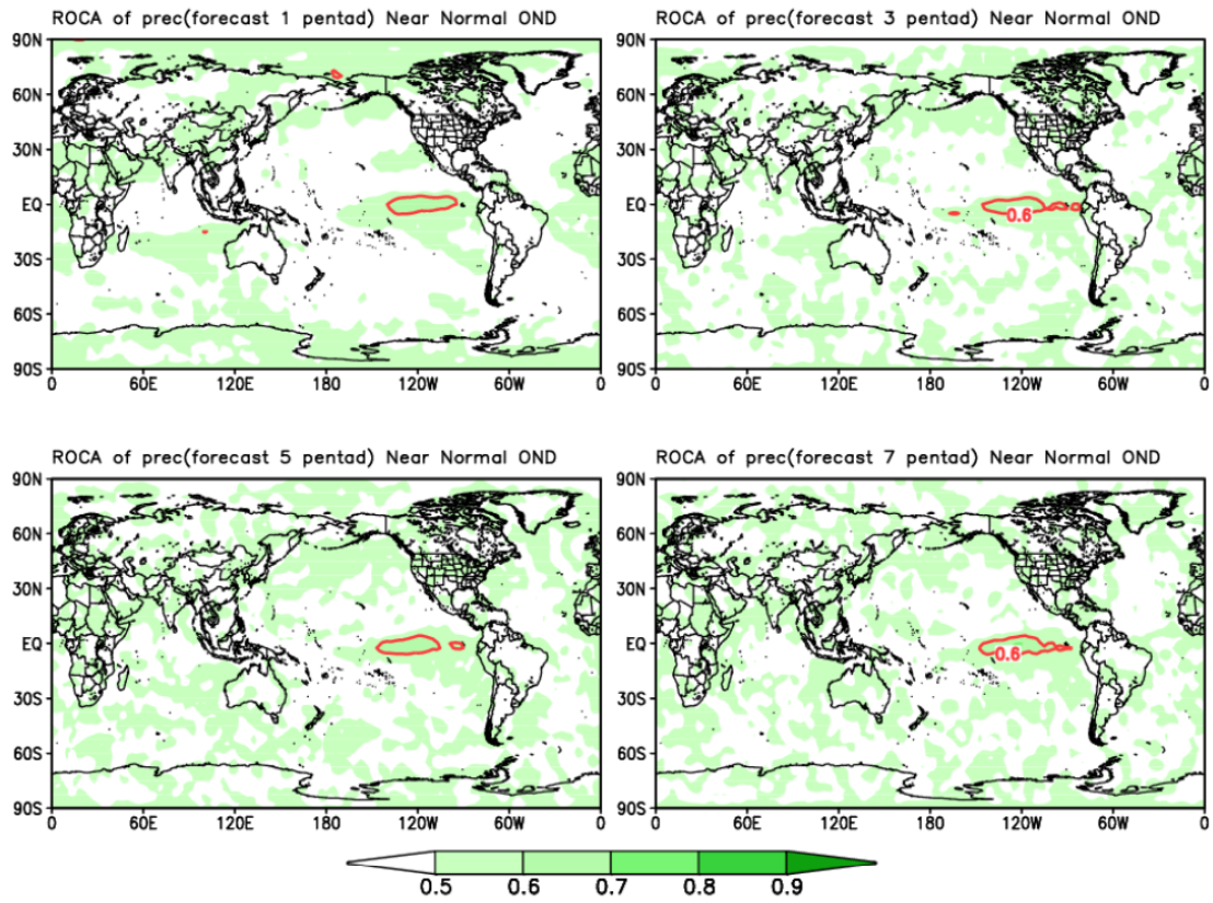
图 47 同图 45, 但为预报降水正常事件
