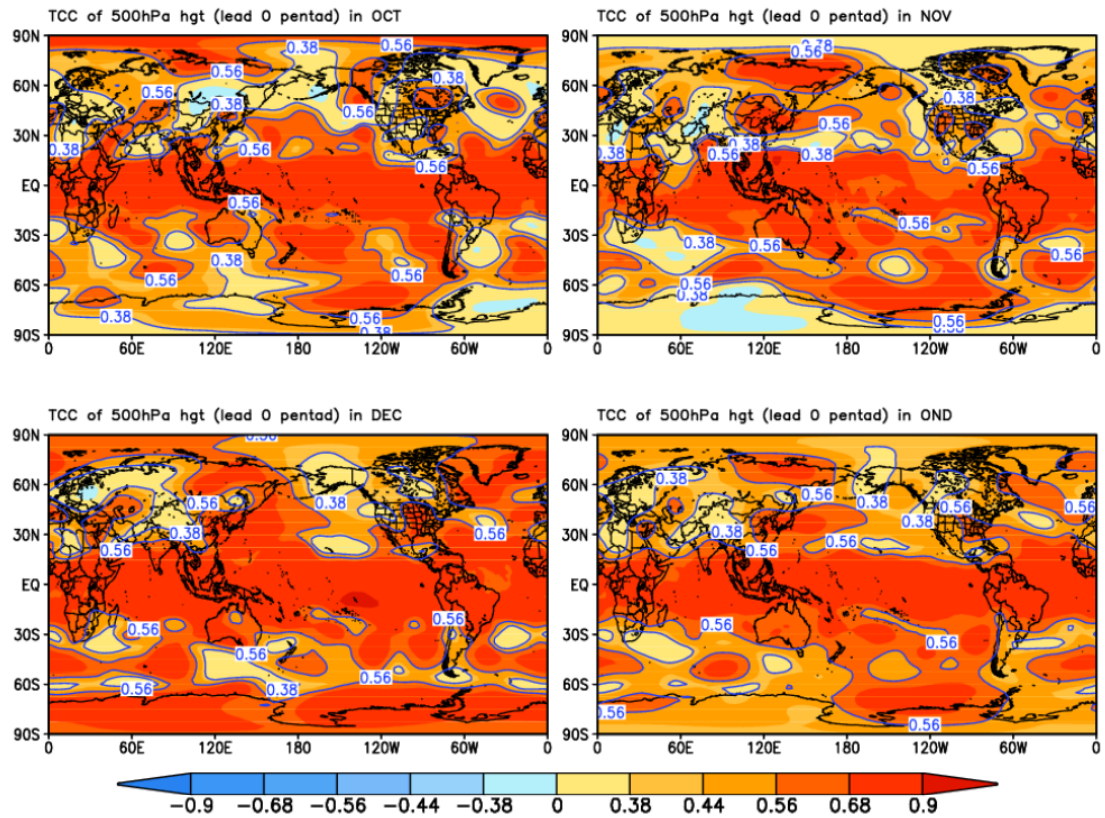
图 26 DERF2.0 超前 0 候起报的全球 10 月、11 月、12 月和第 4 季度的 500hPa 位势高度 (HGT) 的时间距平相关系数 (TCC) 分布, 等值线标定分别代表通过 0.1 和 0.01 显著性检验
