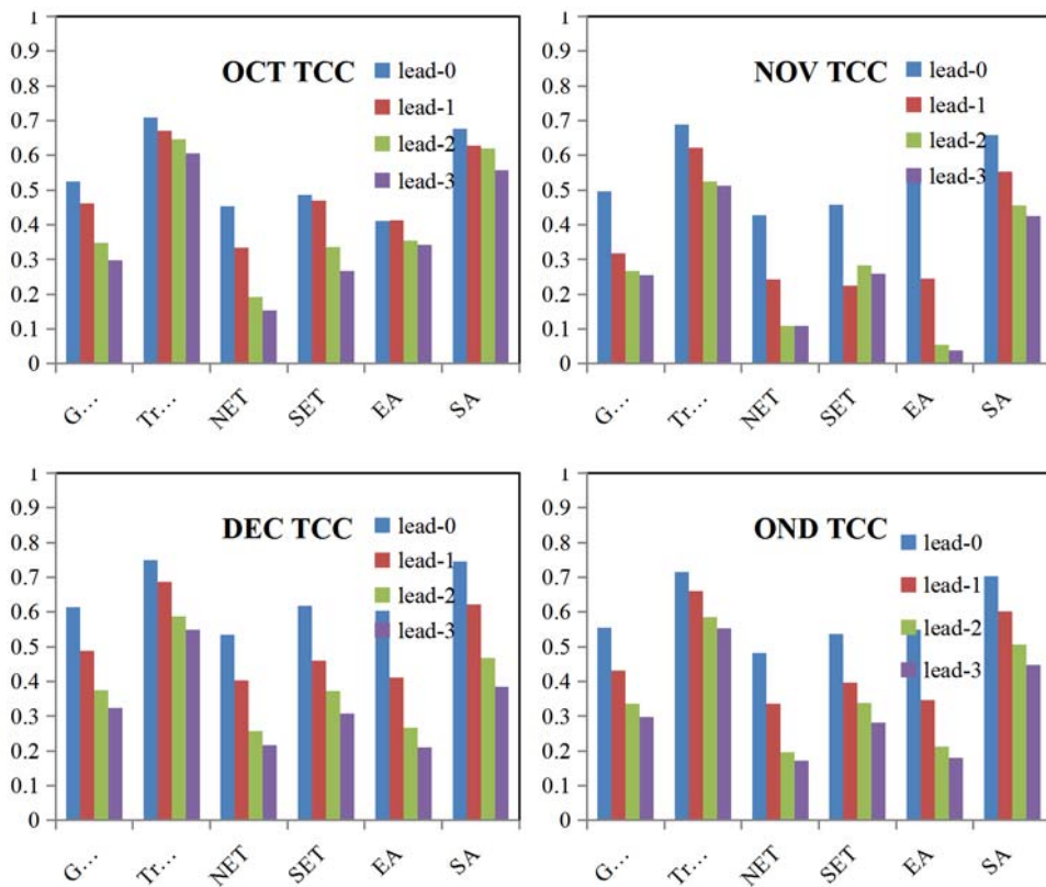
图 27 DERF2.0 在不同 lead time 起报的 10 月、11 月、12 月和第 4 季度的 500hPa 位势高度 (HGT) 的时间
