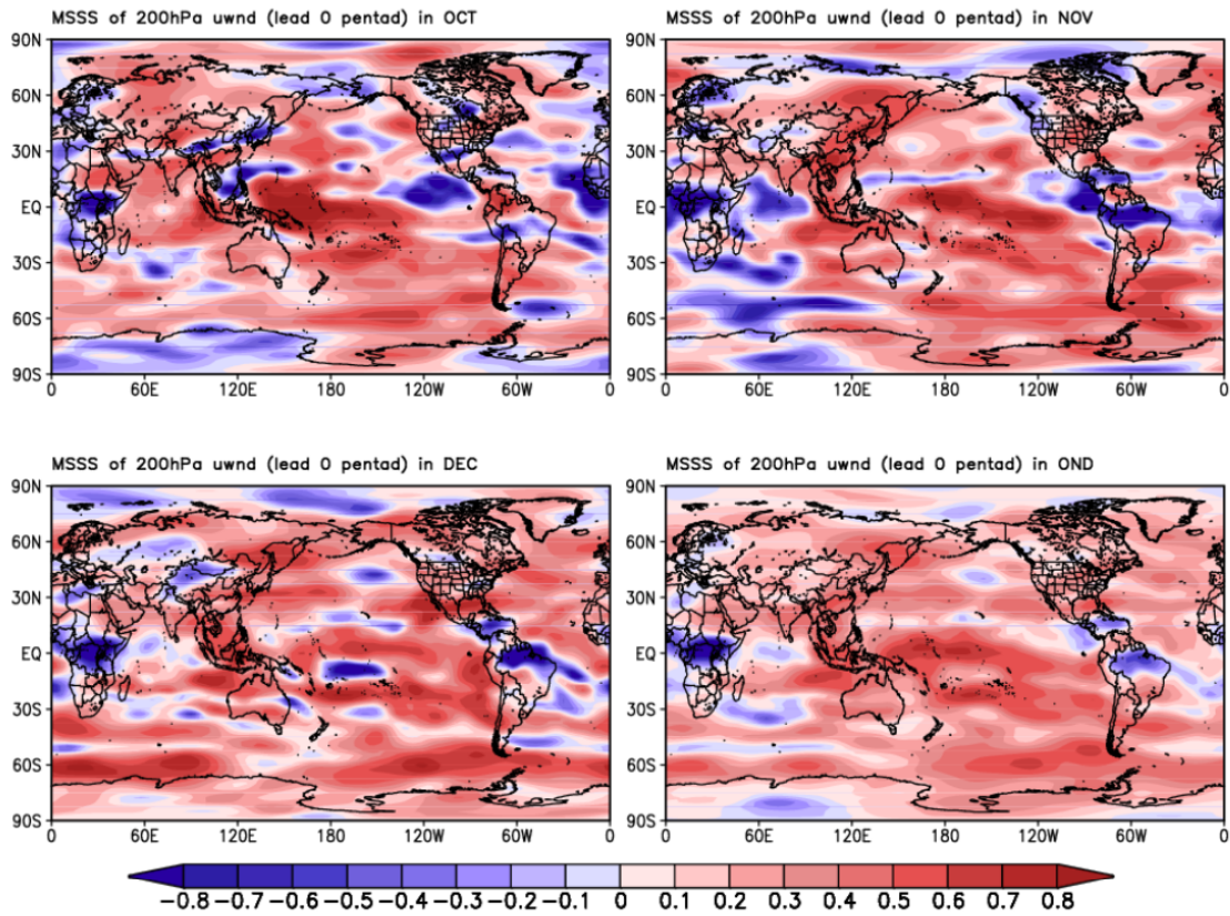
图 34 DERF2.0 超前 0 候起报的全球 10 月、11 月、12 月和第 4 季度的 200hPa 纬向风的平均方差技巧(MSSS) 分布
