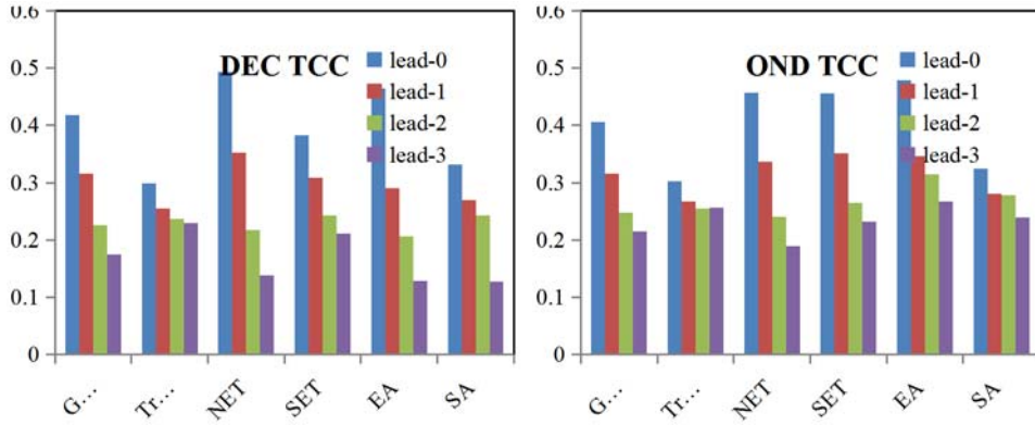
图 10 DERF2.0 在不同 lead time 起报的 10 月、11 月、12 月和第 4 季度的 2m 温度 (t2m) 的时间距平相关系数 (TCC) 在不同地区的平均
