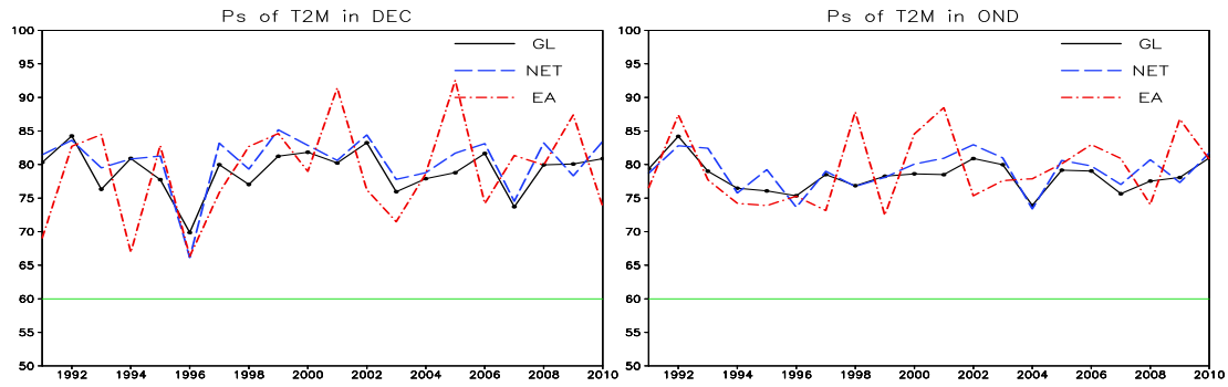
图5 同图2，但为趋势异常综合检验（Ps 评分）逐年演变
