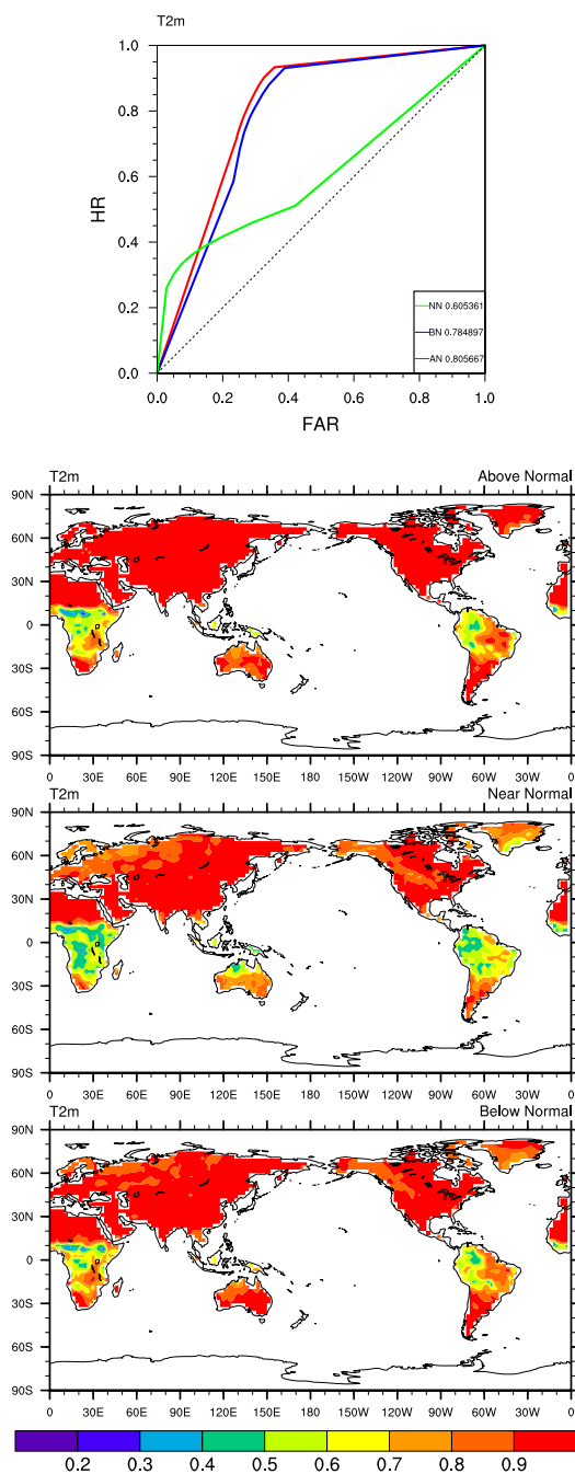
图 37 1991-2010 年 10-12 月 2m 温度 ROC 曲线和 ROCA 面积指数
