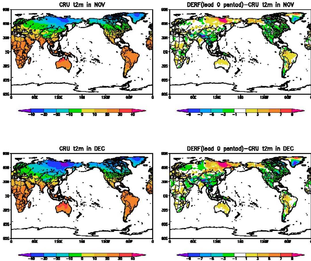
图1 全球多年 (20a) 平均的陆地 10 月、11 月、12 月的 2m 温度 (t2m), 左列为 CRU 观测, 右侧为 DERF (超前 0 候预报) 与观测的差值图
