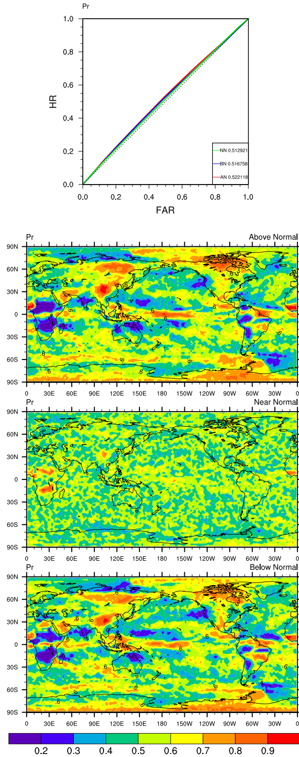
图 38 1991-2010 年 10-12 月降水 ROC 曲线和 ROCA 面积指数
