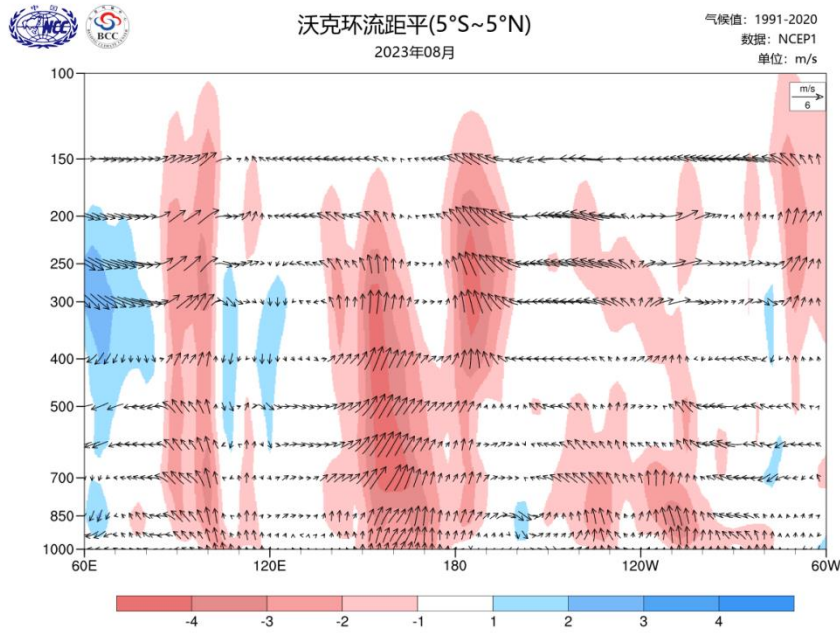
图5 2023年8月赤道(5°S-5°N)平均垂直高度-经度环流距平剖面图
