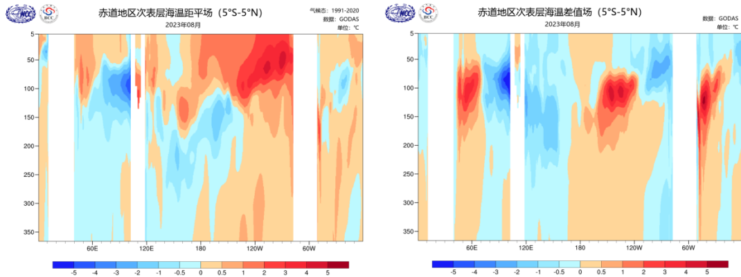
图3 2023年8月赤道印度洋-太平洋次表层海温距平深度-经度剖面（左） 及其与上月差值分布（右）（℃）
