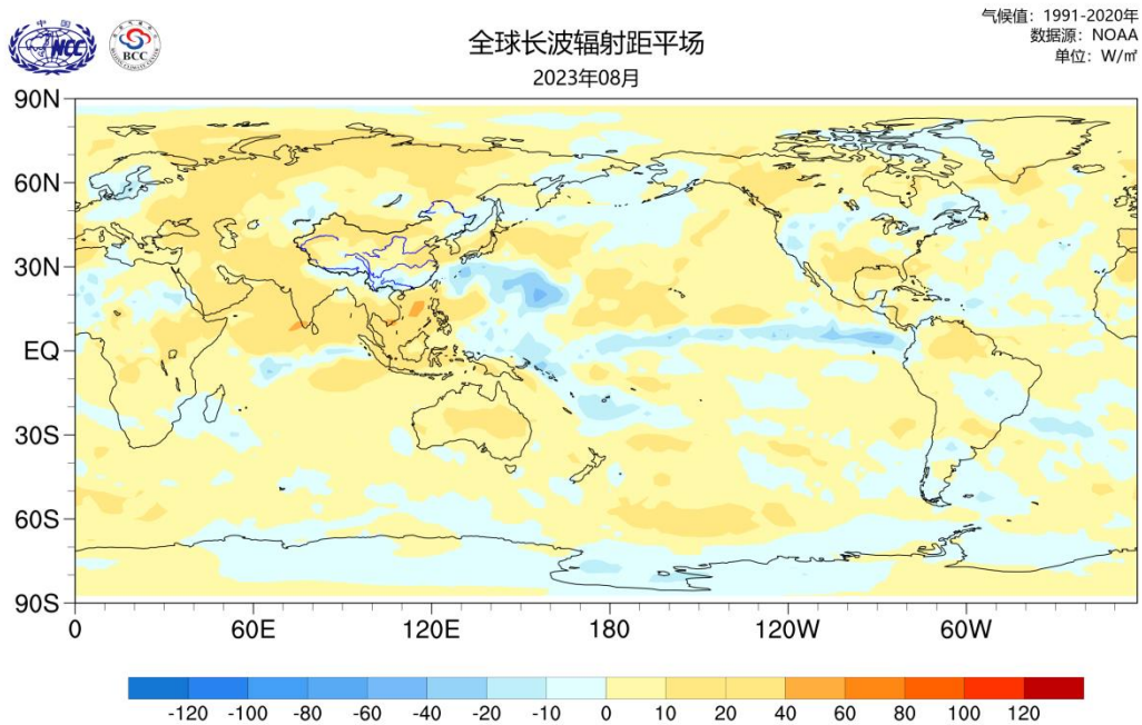
图4 2023年8月平均射出长波辐射（OLR）距平图（ W/m^2 ）
