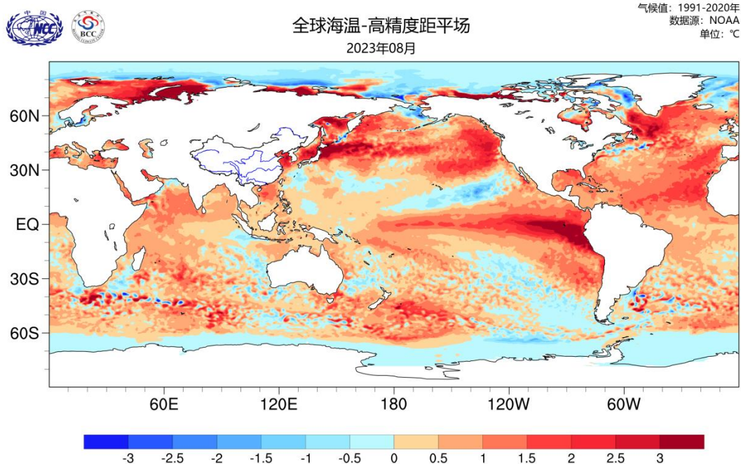
图 1 2023 年 8 月海表温度距平分布图 ( ^{\circ}\text{C} )
