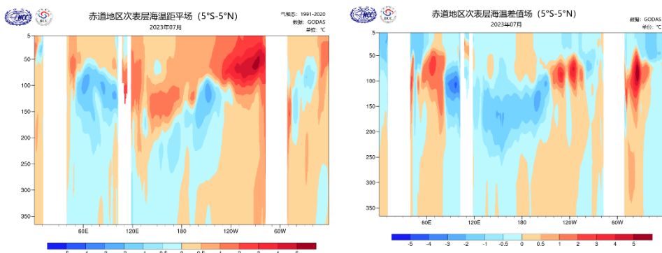
图3 2023年7月赤道印度洋-太平洋次表层海温距平深度-经度剖面(左)
