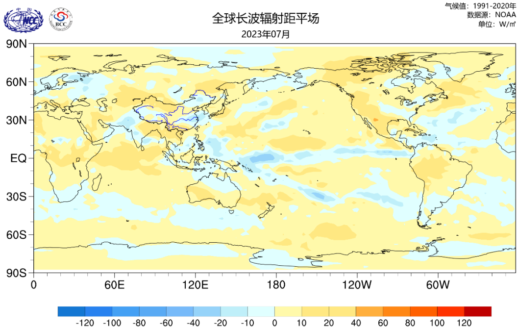
图4 2023年7月平均射出长波辐射（OLR）距平图（W/m 2 ）
