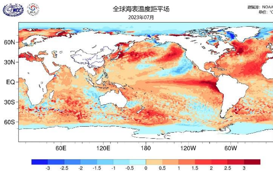
图 1 2023 年 7 月海表温度距平分布图 ( ^{\circ}\text{C} )
