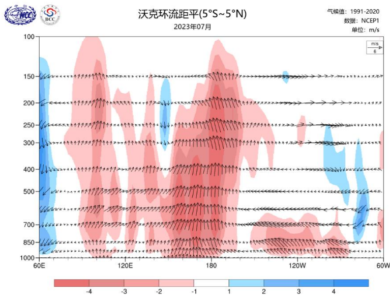
图5 2023年7月赤道(5°S-5°N)平均垂直高度-经度环流距平剖面图 (阴影区表示垂直速度距平, 单位 0.01Pa/s)
