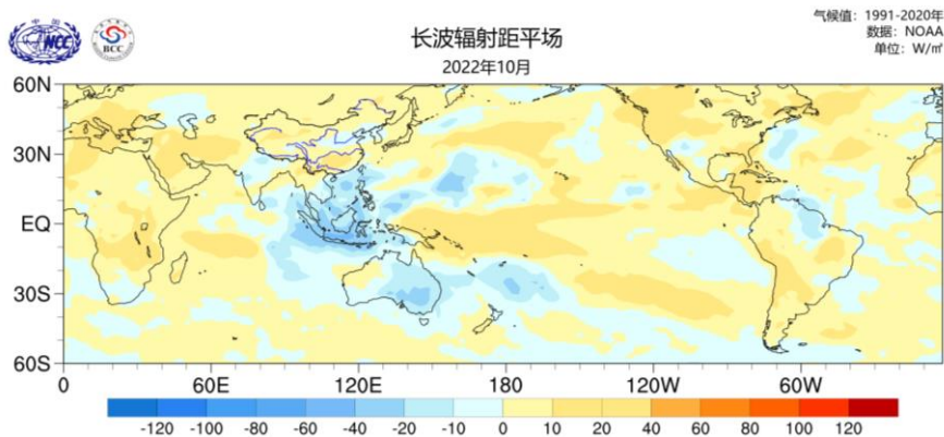
图4 2022年10月平均射出长波辐射量（OLR）距平图（W/m 2 ）
