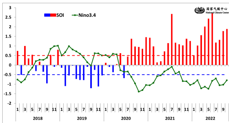
图 2 Niño3.4 区海温指数 ( ^{\circ}\text{C} ) 和 SOI 指数逐月演变
