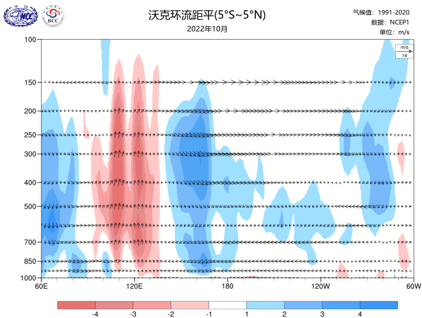
图5 2022年10月赤道（5°S-5°N）平均垂直-经度环流距平剖面图 （阴影区表示垂直速度距平，单位 0.01Pa/s）
