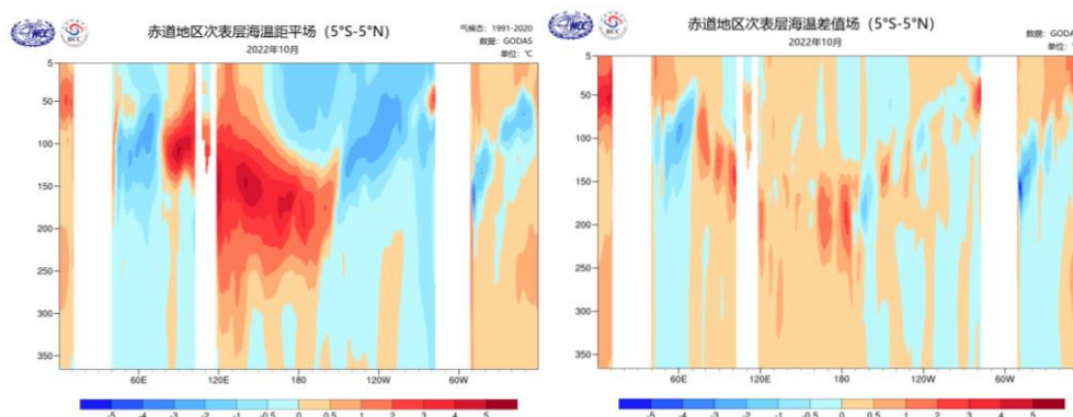
图3 2022年10月赤道印度洋-太平洋次表层海温距平深度-经度剖面（左）及其与上月差值分布（右）（ ^{\circ}\text{C} ）
