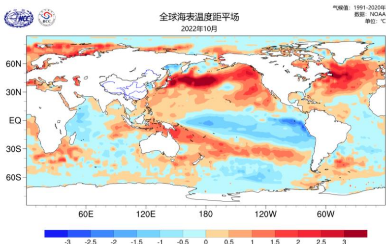
图 1 2022 年 10 月海表温度距平分布图 ( ^{\circ}\text{C} )
